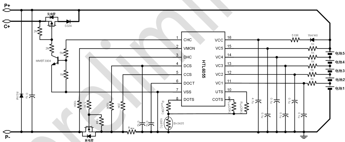
图3 5节电池包的P型充电管和N型放电管的C+分口典型应用电路图
