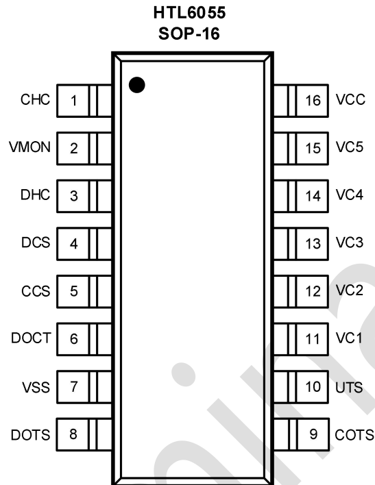
图 4 引脚分布
