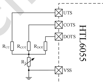
图 6 温度保护外围电路
