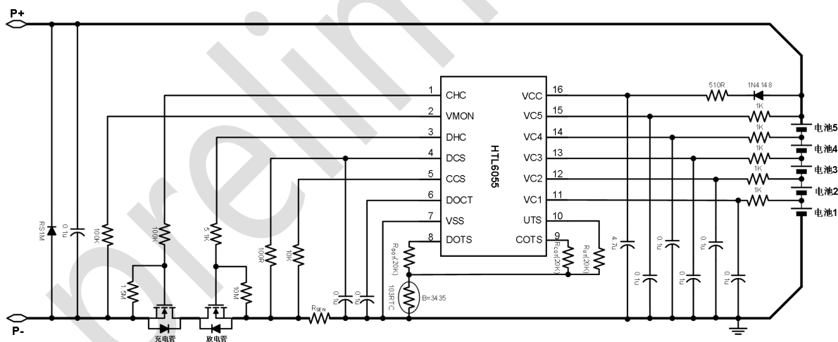
图1 5节电池包的N型充电管和N型放电管的同口典型应用电路图
