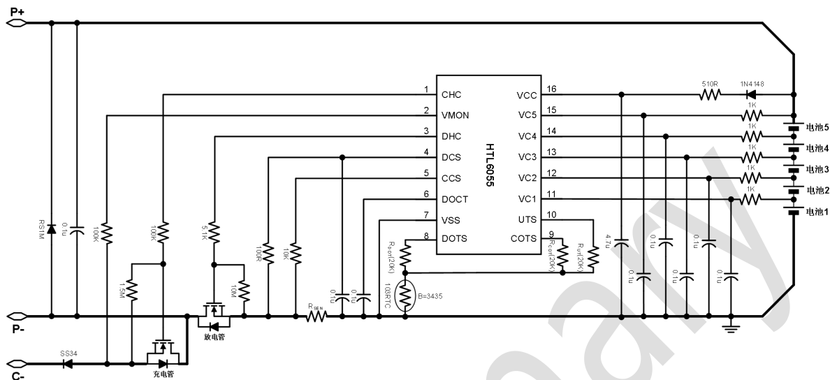
图 2 5 节电池包的 N 型充电管和 N 型放电管的 C-分口典型应用电路图
